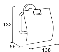
# 740038 Papierrollenhalter Toilet Roll Holder
