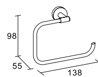
# 740007 Papierrollenhalter Toilet Roll Holder # 740066 Ausführung links Left hand mount
